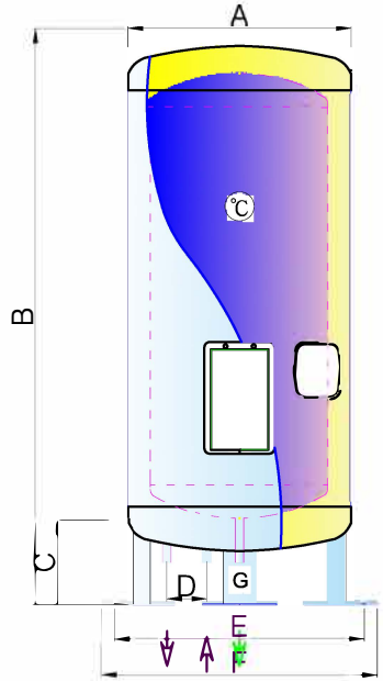
立地式 電熱水器尺寸圖
