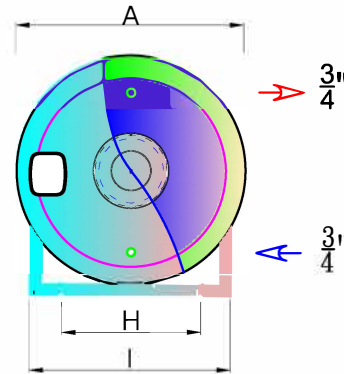
側視圖
