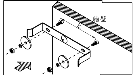
掛壁式：掛耳壁虎裝置圖說
