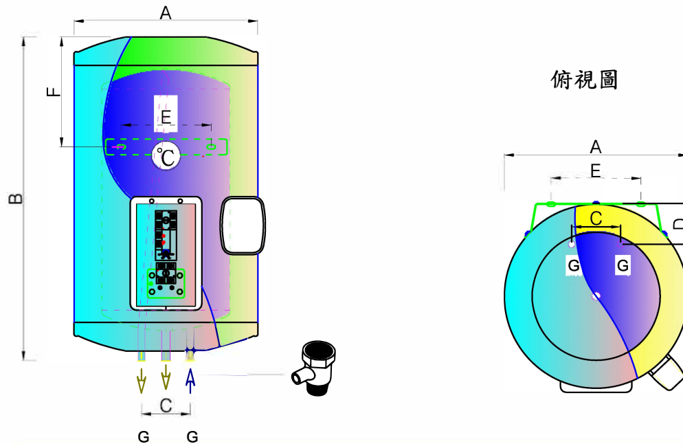
掛壁式 電熱水器尺寸圖
