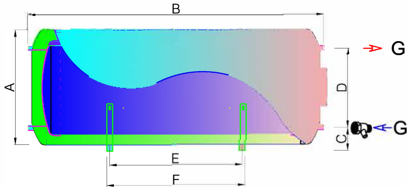
臥地式 電熱水器尺寸圖
